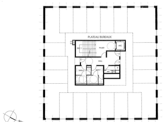
NIVEAU 2 à 4 - ECHELLE : 1/100
