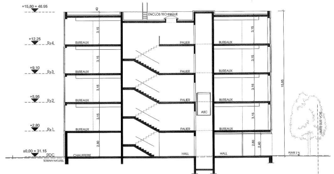
COUPE DE PRINCIPE - ECHELLE : 1/100
